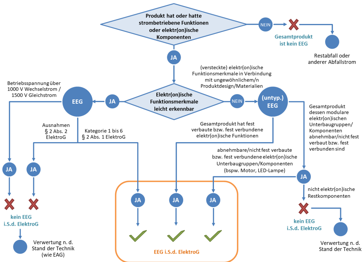
Abbildung 3: Entscheidungsbaum für die Identifikation von „untypischen“ Elektro- und Elektronikgeräte (EEG).
